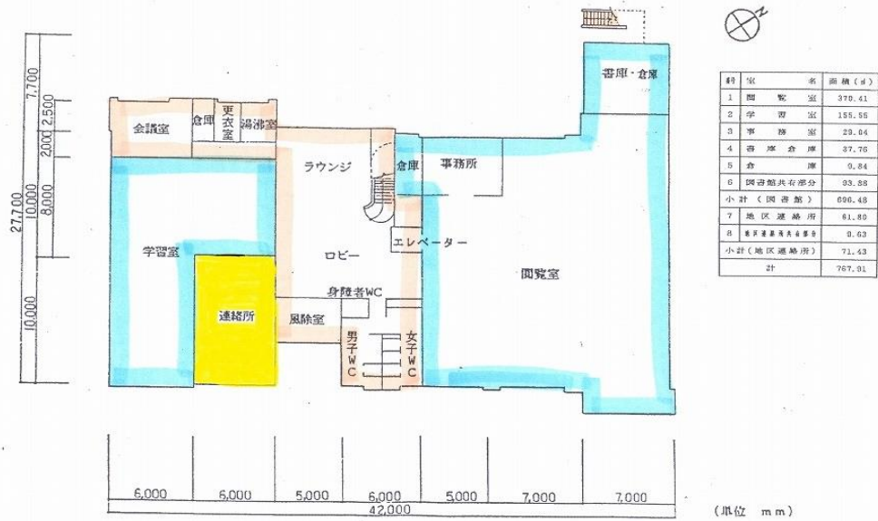
1階 平面図
