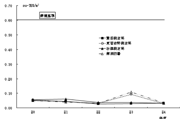
図 3.10.1 ダイオキシン類大気環境調査結果の年平均推移水質
