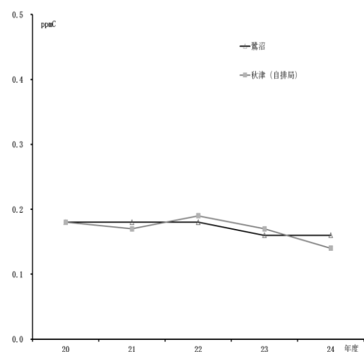
図 3.6.5 非メタン炭化水素経年変化
