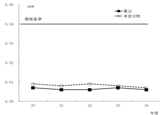
図 3.6.2 二酸化硫黄経年変化
