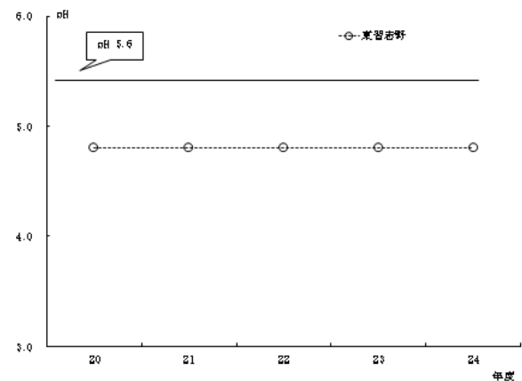
図 3.6.6 酸性雨 pH 年間平均値
