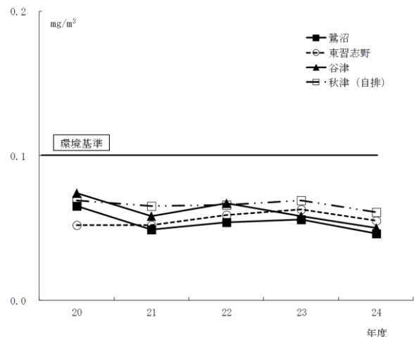
図 3.6.4 浮遊粒子状物質経年変化
