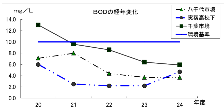
図 3.7.2 河川 3 地点の BOD の経年変化(75%値)
