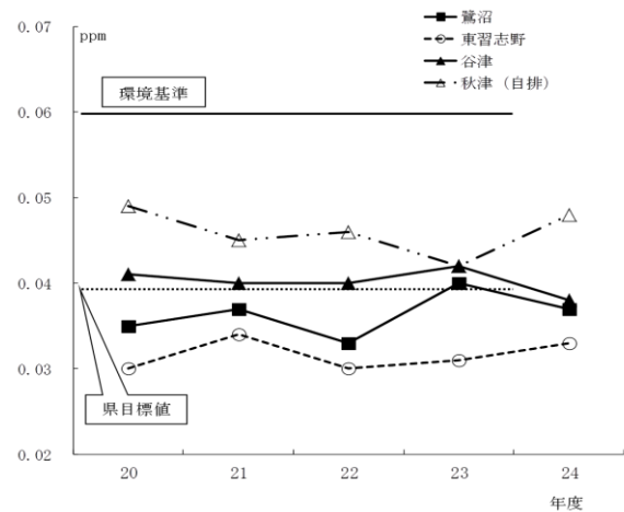
図 3.6.3 二酸化窒素経年変化
