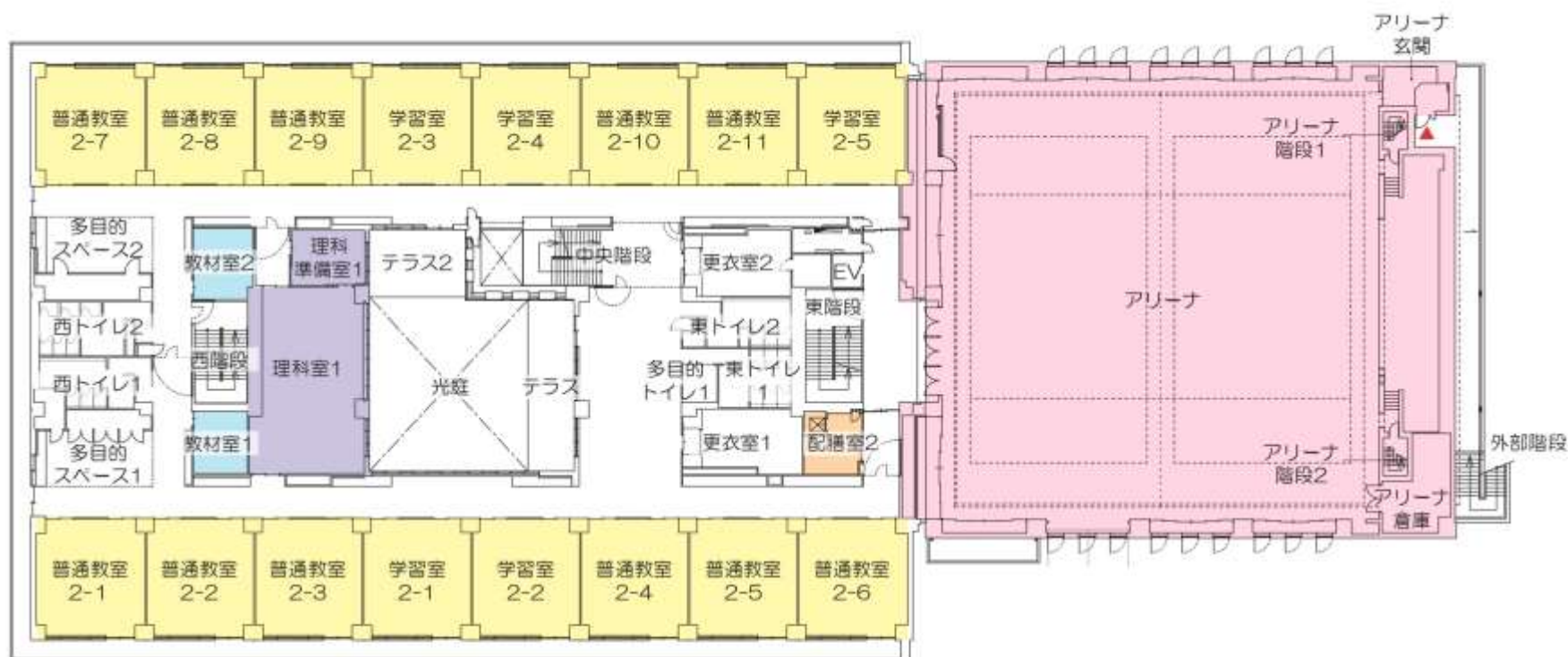
2階 平面図
