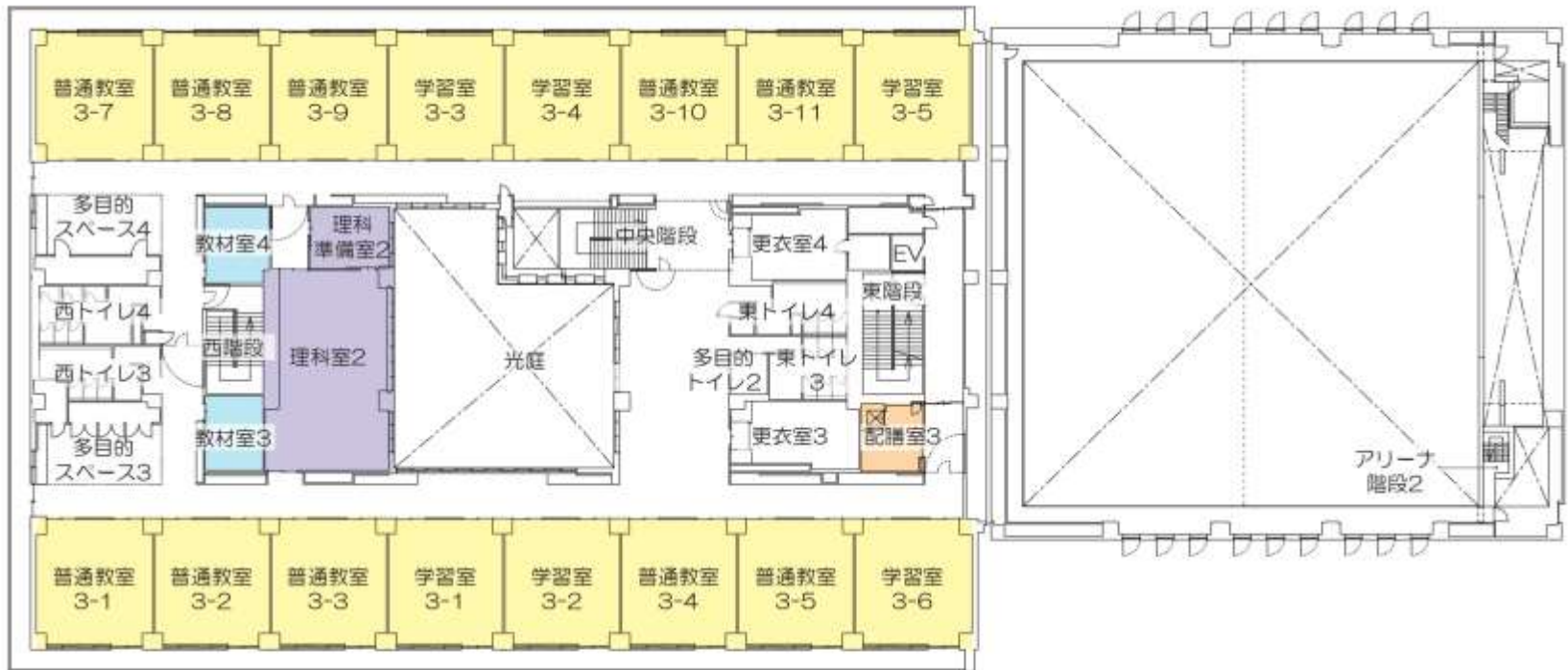
3階 平面図
