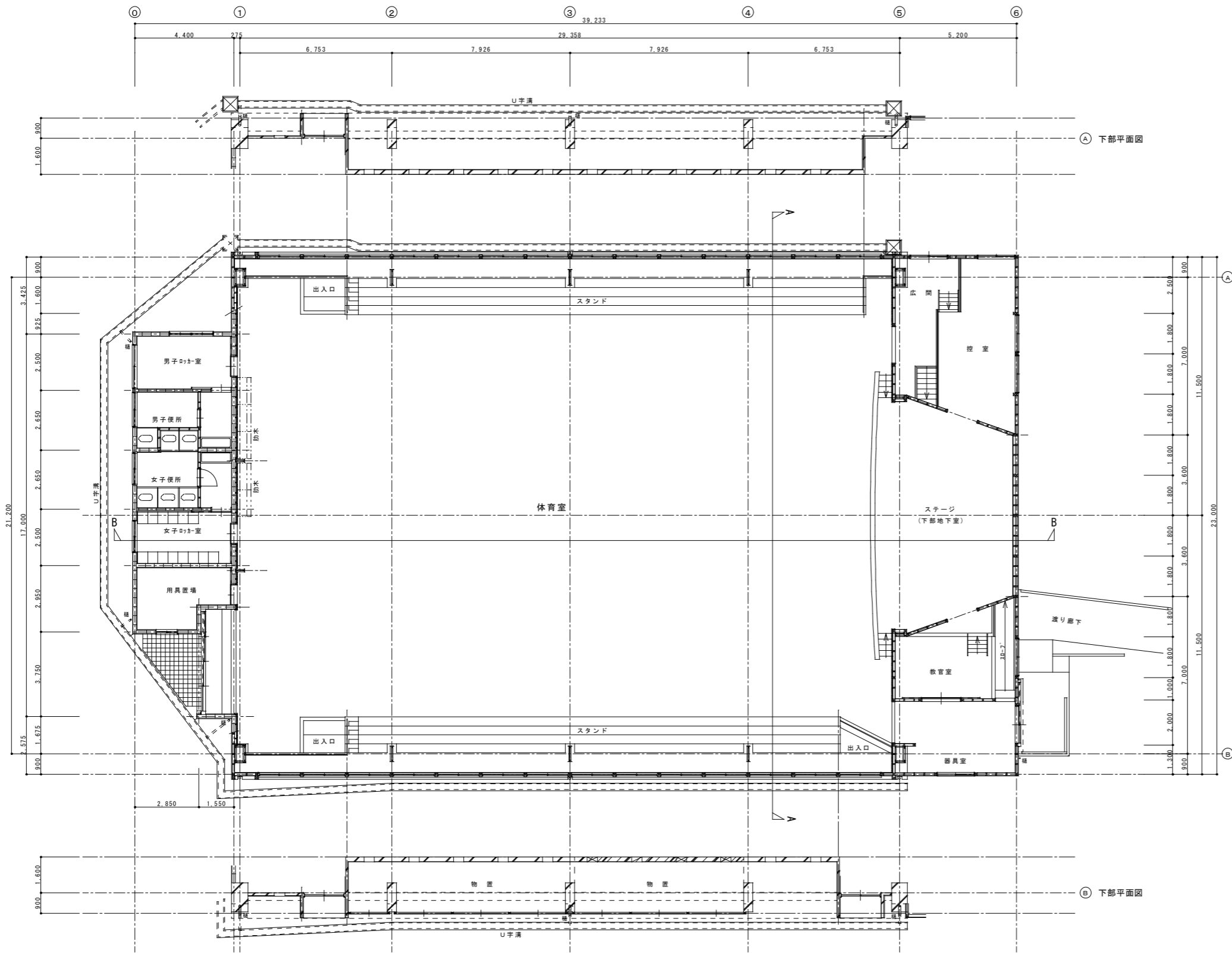
1階平面図
