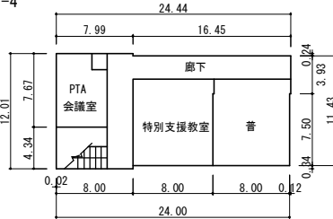
3階 平面図
