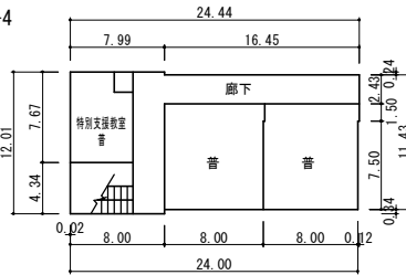
3階 平面図
