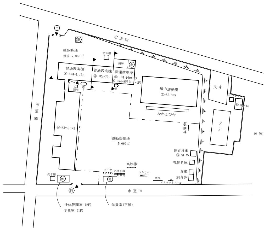
配 置 図
