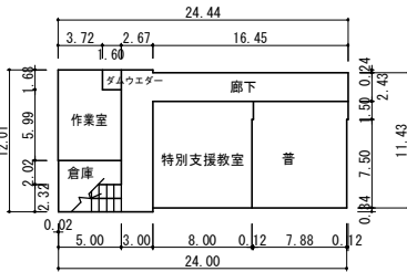
1階 平面図
