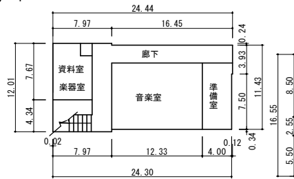
4階 平面図
