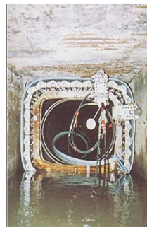
管渠耐震化工法(更生工法の採用)
