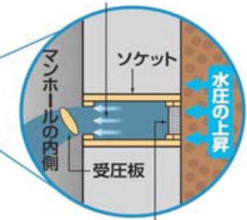
マンホール耐震化工法
