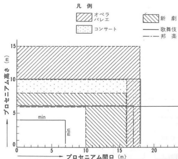
■オーデトリウム目的によるプロセニウム開口寸法 出典：『建築計画チェックリスト 集会・催し施設』彰国社編(1981)
