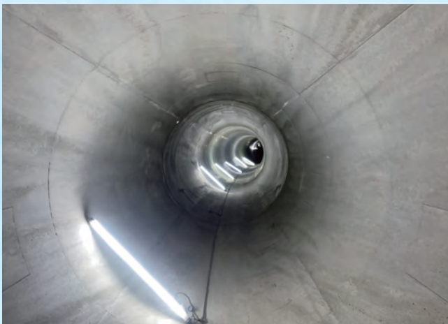
📷3 第3工区のカーブで撮影した写真です。コンクリート打設時、スチールフォームは通常9mを標準としていますが、カーブに合わせて3m、6m、9mの長さに調整しながら施工します。
