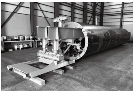
↑スチールフォーム(移動式型枠)全長約9.0m
