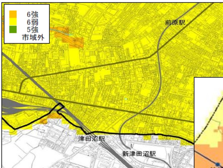
東京湾北部地震（M7.3）震度分布図 （出典：船橋市地区別防災カルテ）
