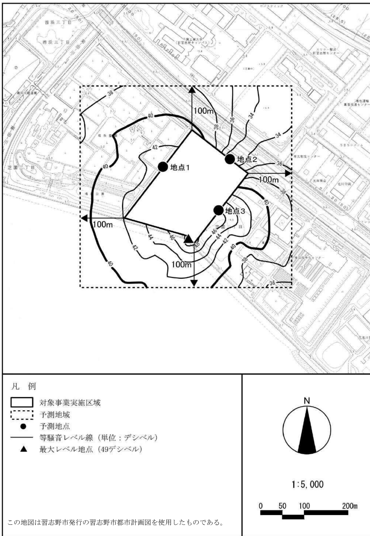
図 7-2-3.10(2) 施設の稼働による騒音予測結果 (朝・夕・夜間)
