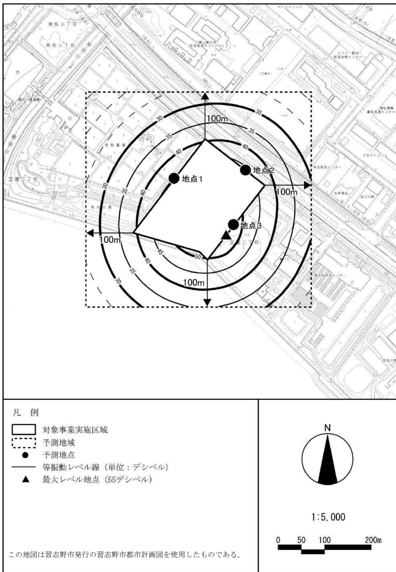
図 7-2-4.3 建設機械稼働による振動予測結果
