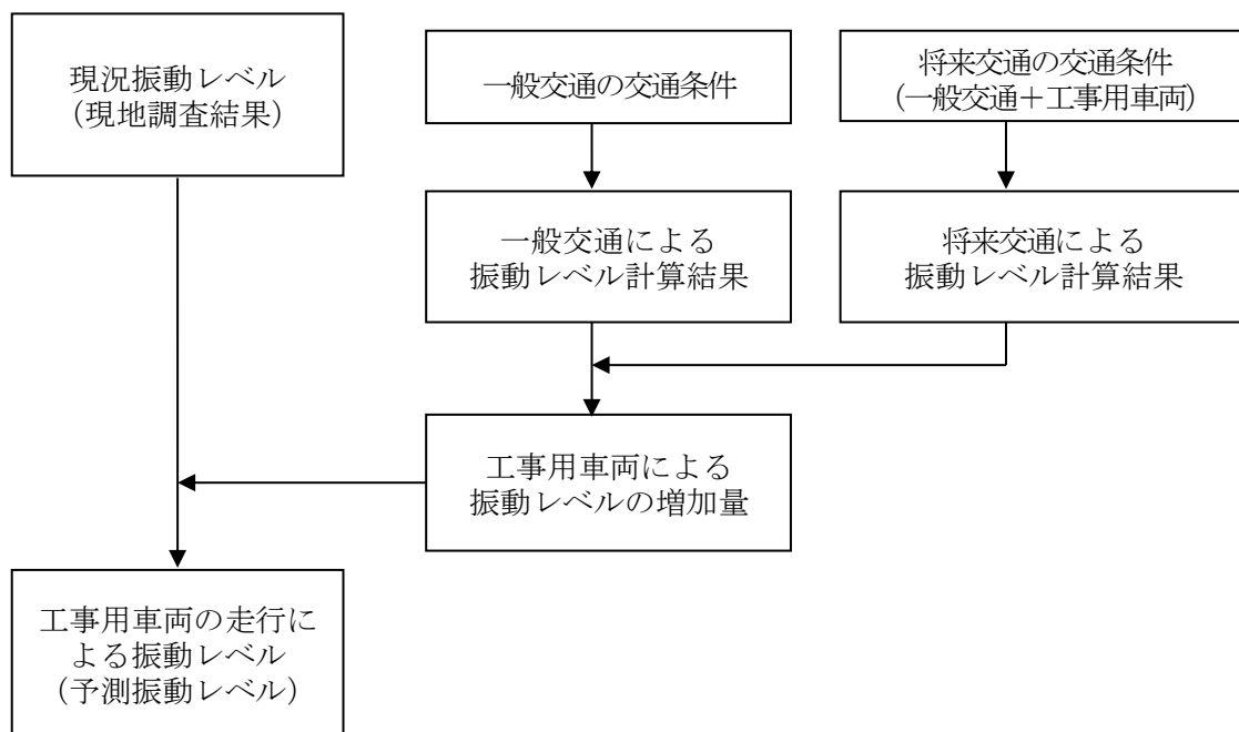
図 7-2-4. 4 工事用車両による道路交通振動の予測手順
