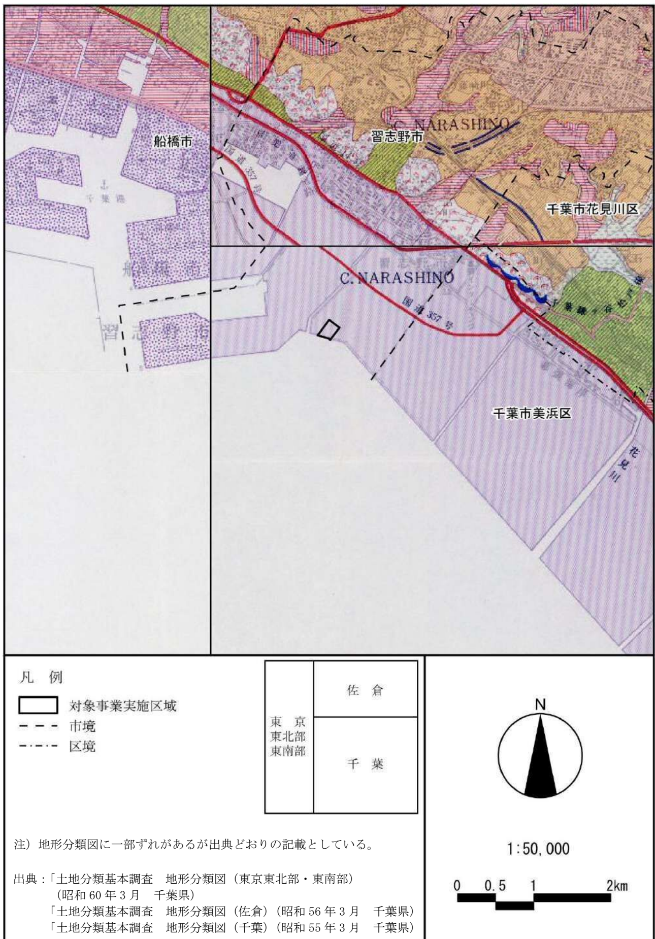
図 3-1-20(1) 地形分類図
