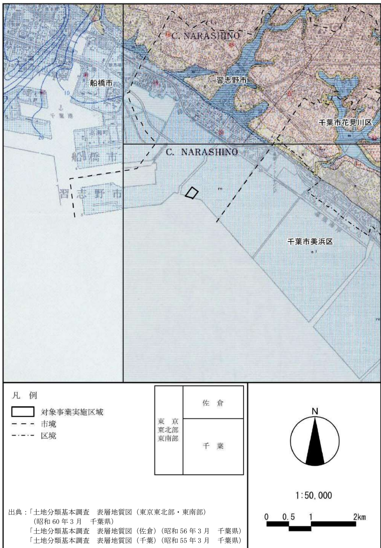
図 3-1-21(1) 表層地質図
