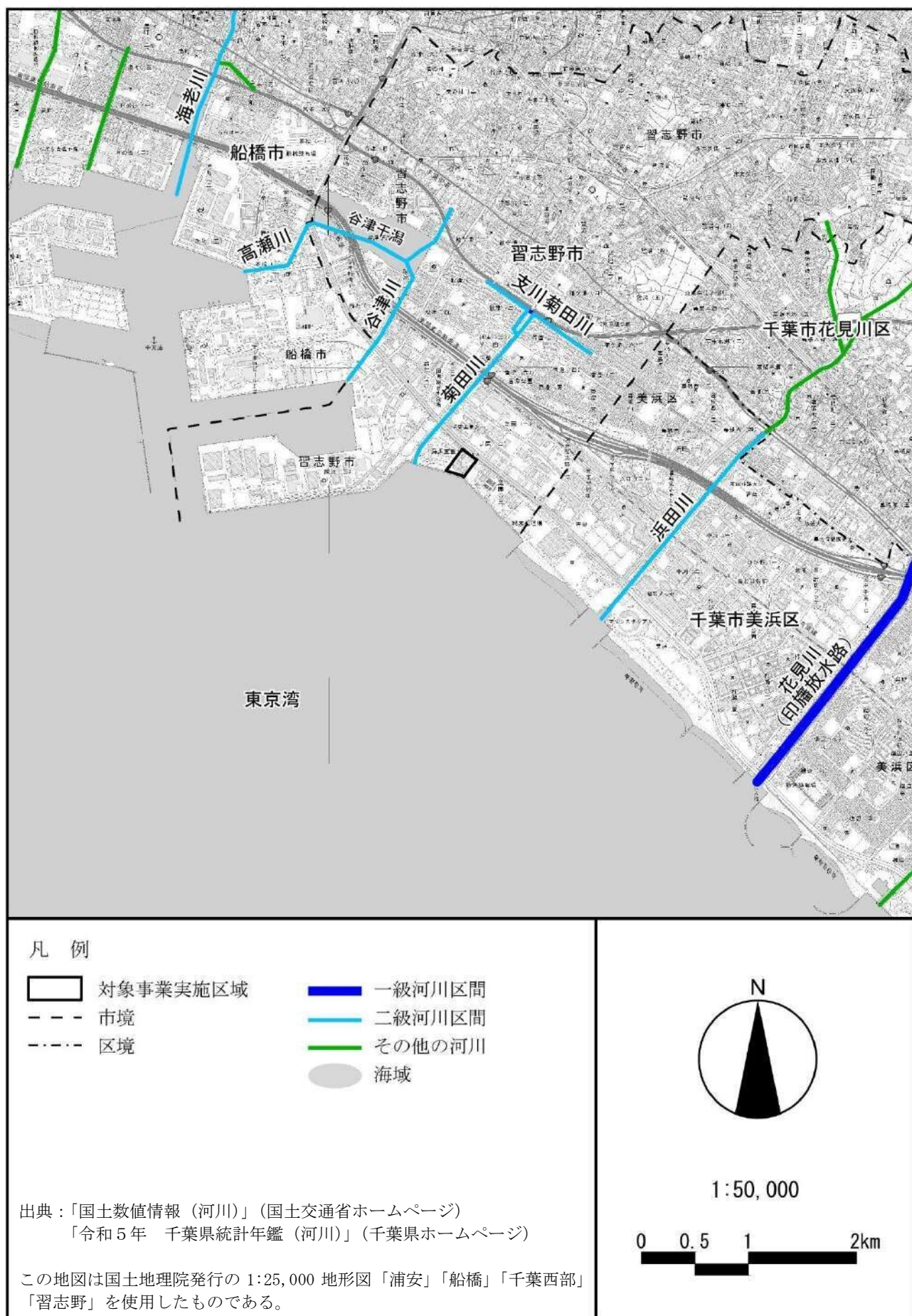
図 3-1-15 水象の状況
