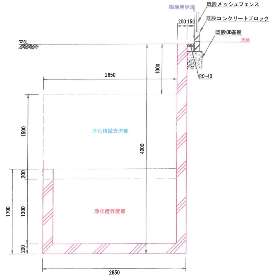
浄化槽B-B'断面図 S=1:30
