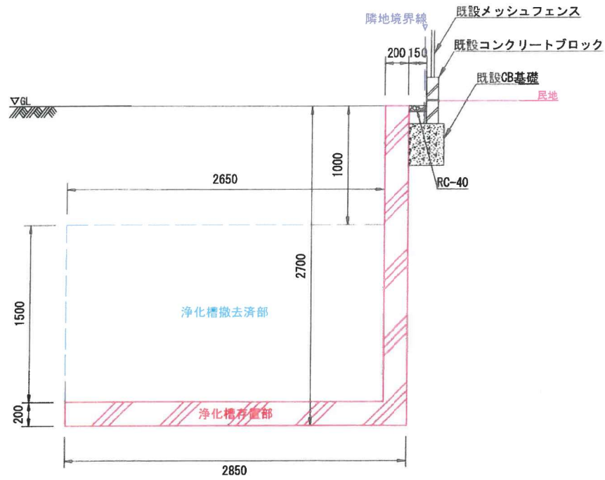
浄化槽A-A'断面図 S=1:30
