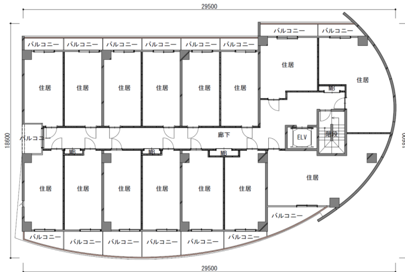
2-3階平面図
