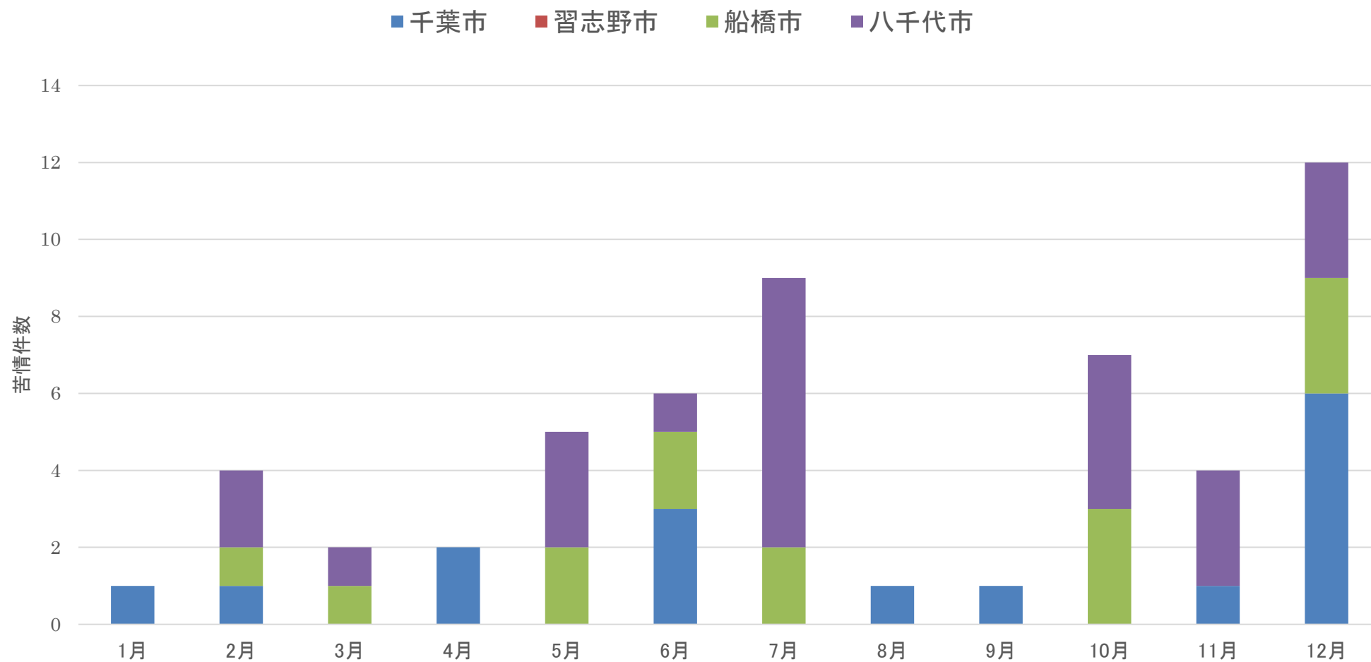
図2 習志野演習場の航空機騒音月別苦情発生状況(平成31年1月～令和元年12月)
