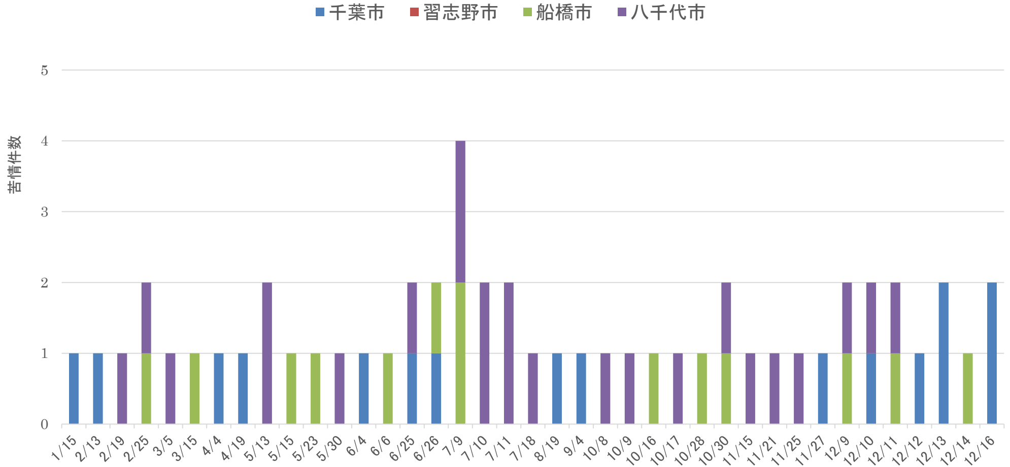
図1 習志野演習場の航空機騒音日別苦情発生状況(平成31年1月～令和元年12月)
