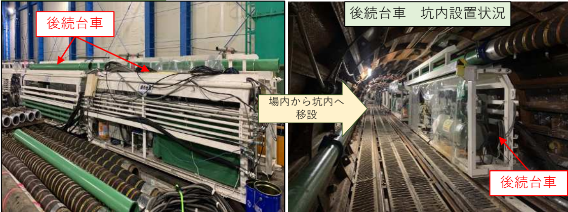
後続台車：シールド掘進に必要な設備を搭載した車
